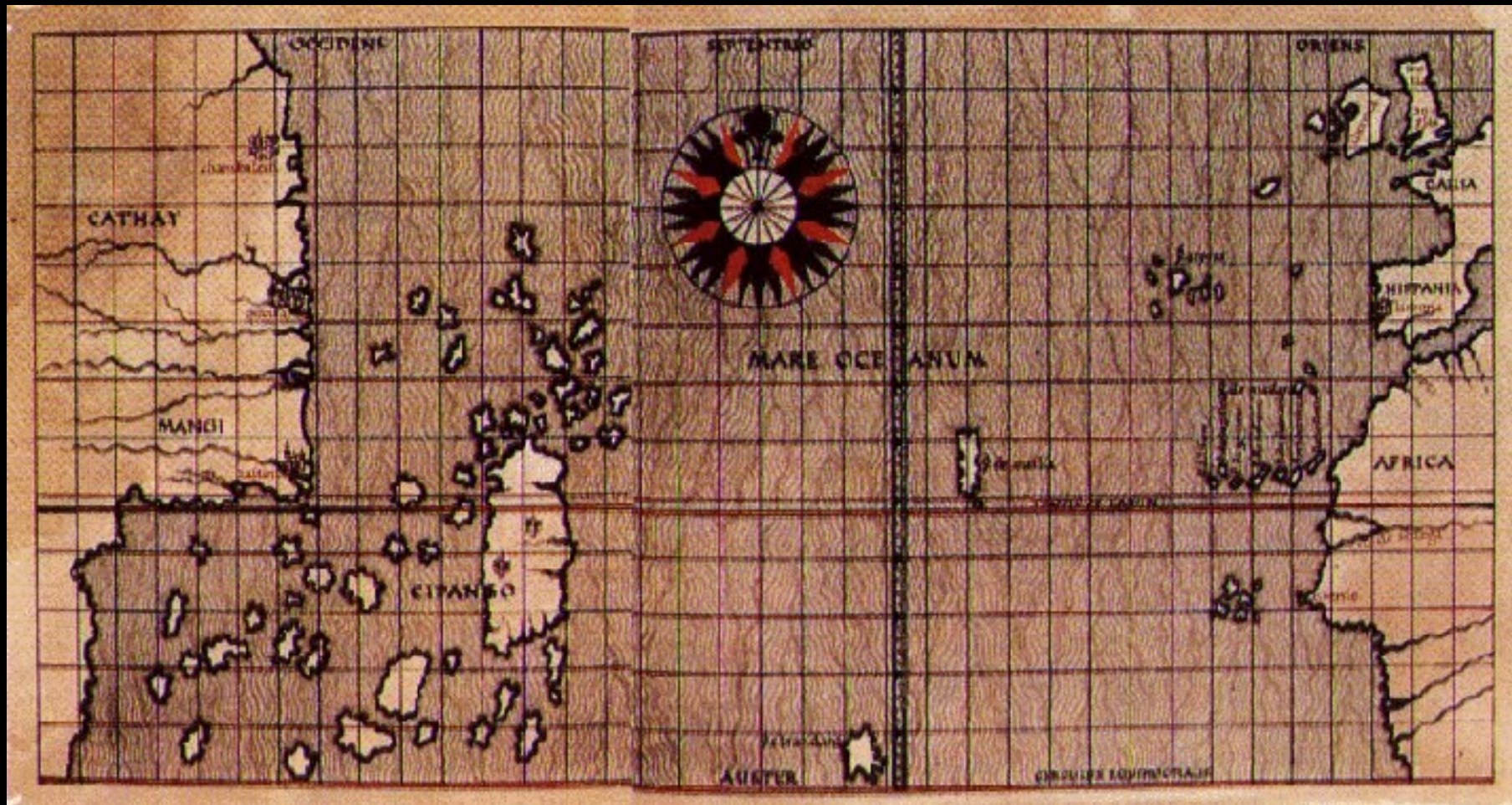
L'Océan Atlantique, d'après Toscanelli, 1468
